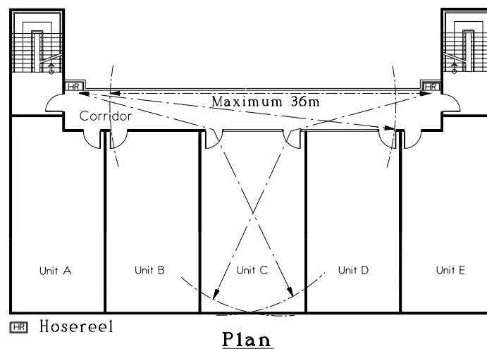
Diagram 6.2.8(d) - 2
