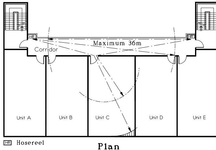
Diagram 6.2.8(d) - 1
