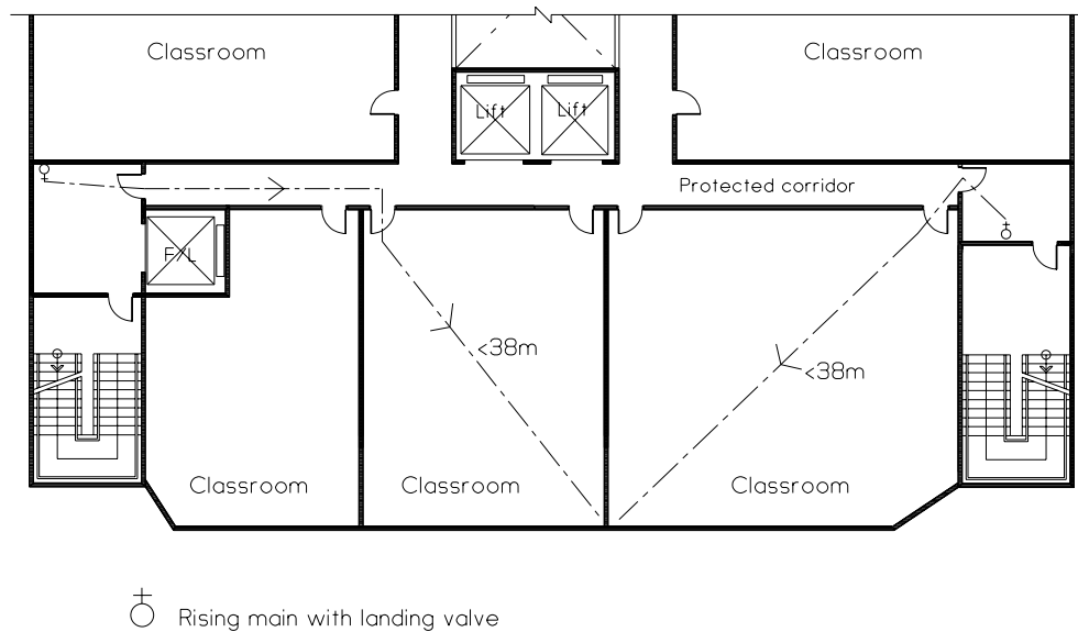
Diagram 6.2.2(d) – 1
