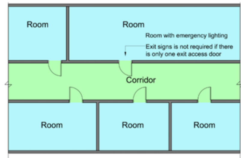
Diagram 8.1.7a.(3)(a)(i)
