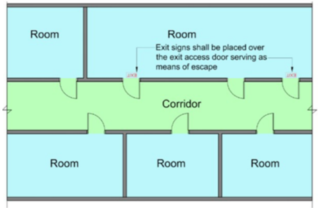
Diagram 8.1.7a.(2)
