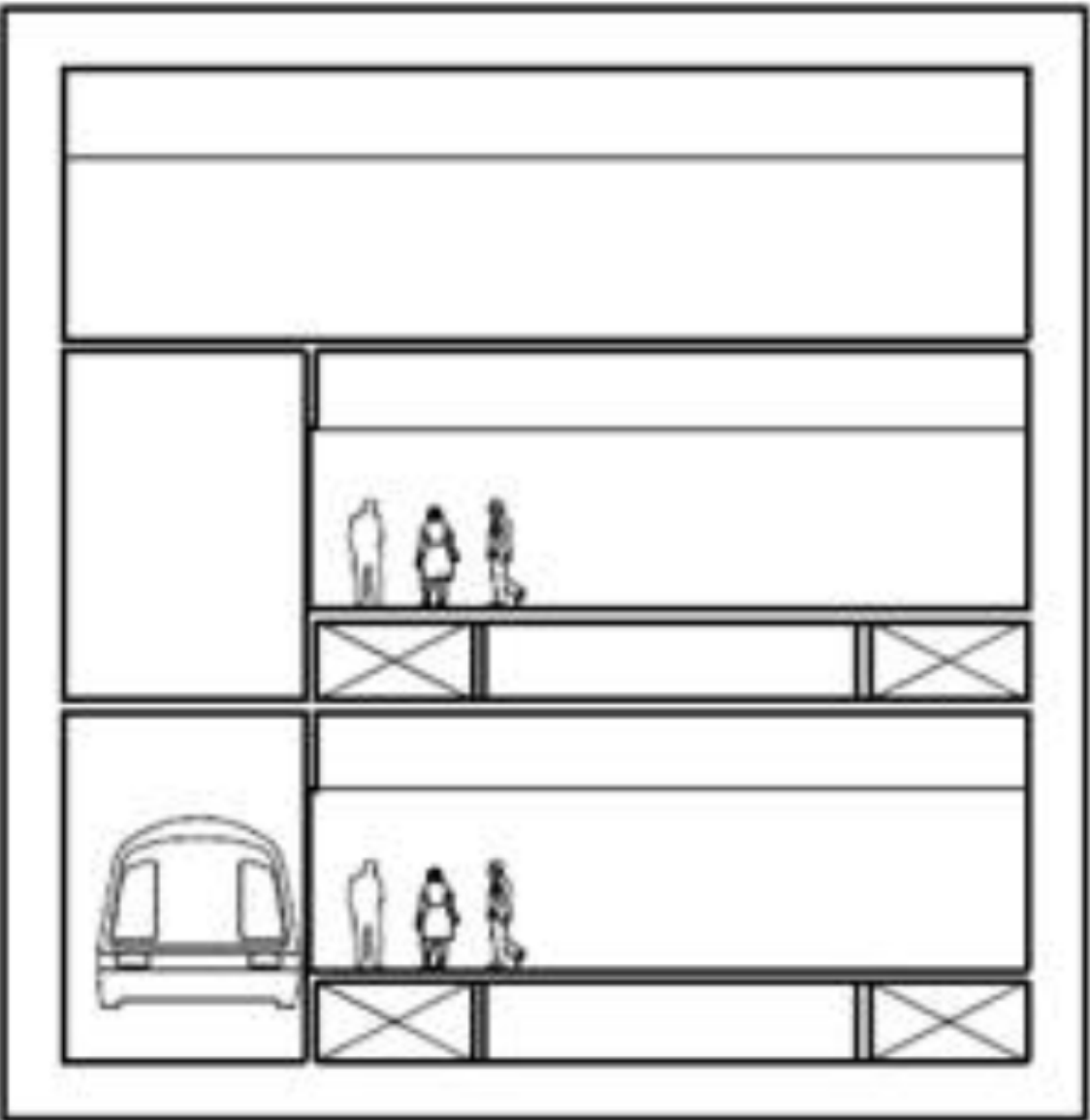
Diagram 2.3.2 – 1
