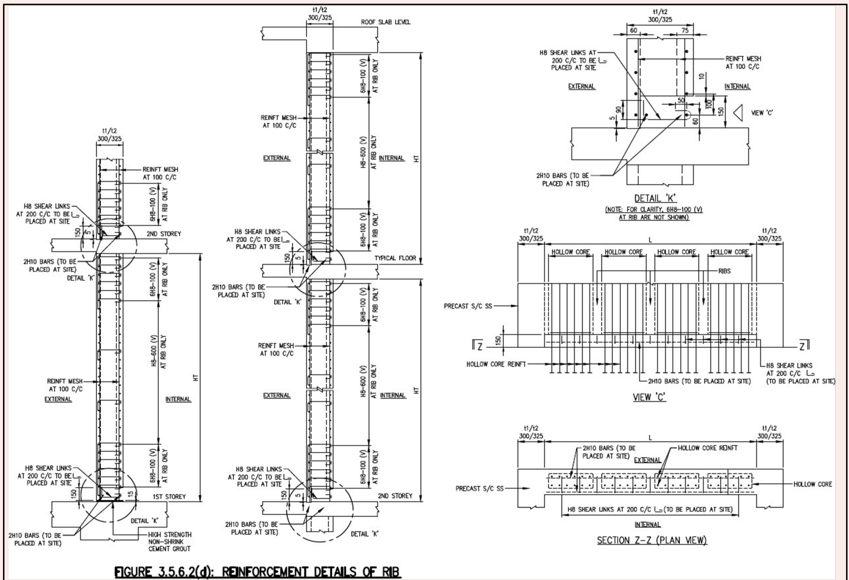
FIGURE 3.5.6.2(d)
