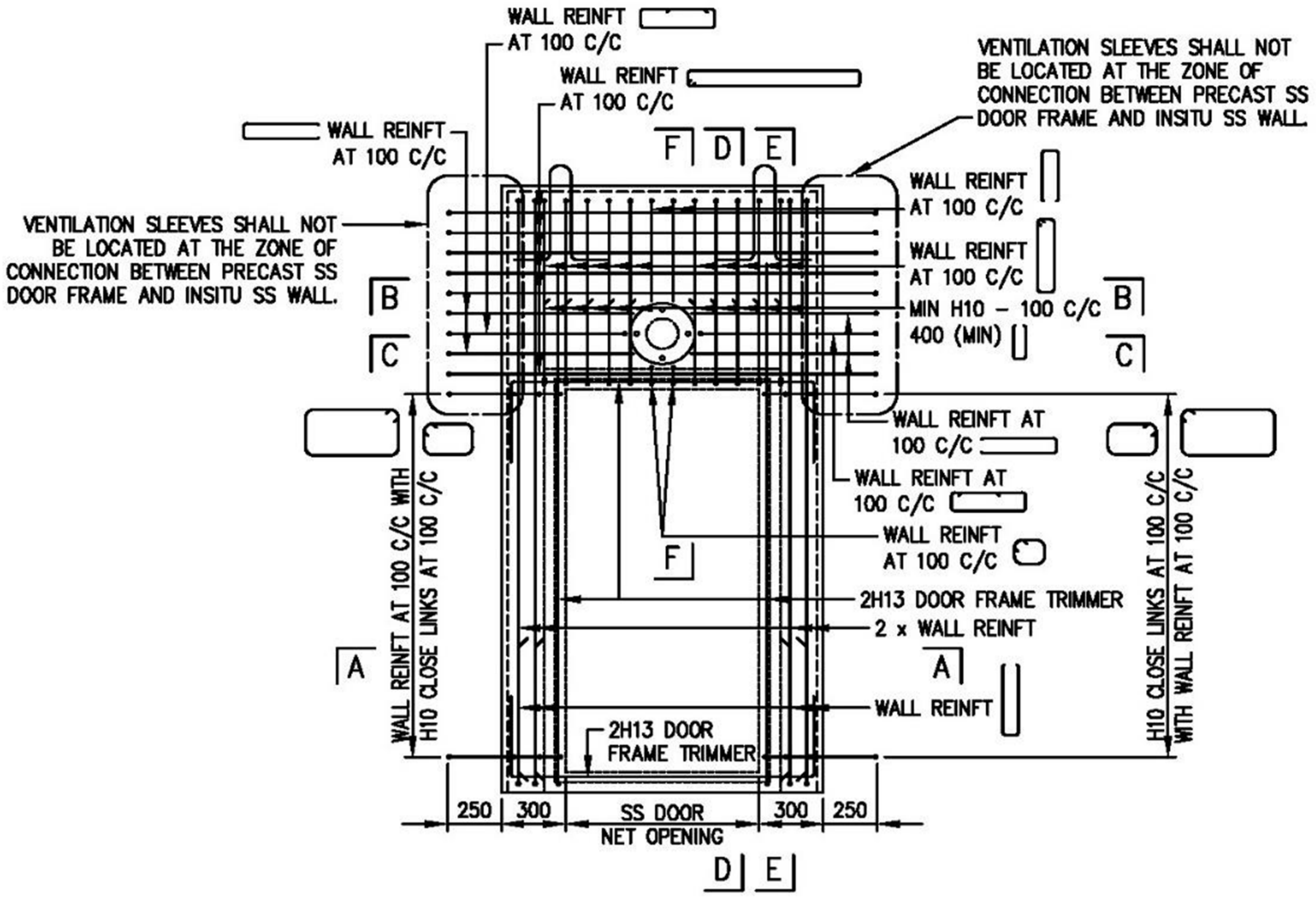
ELEVATION
